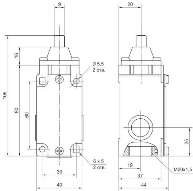
толкатель
